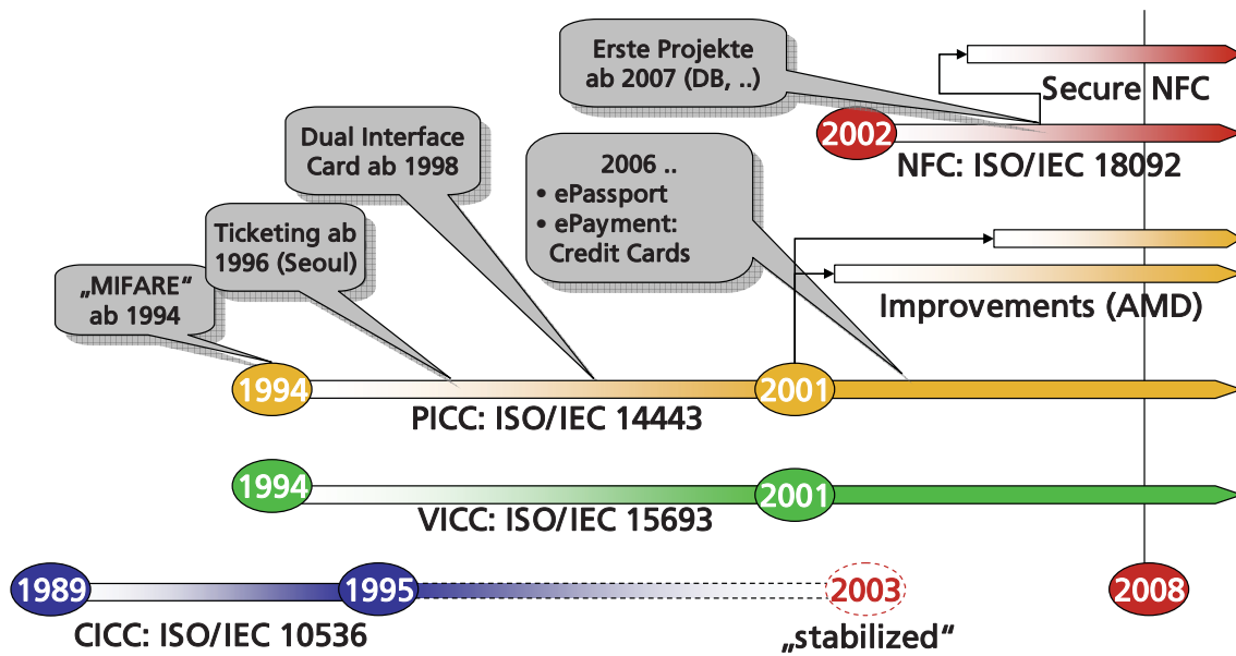
Abbildung 1: Die Zeitskala der Entwicklung kontaktloser Chipkarten.
